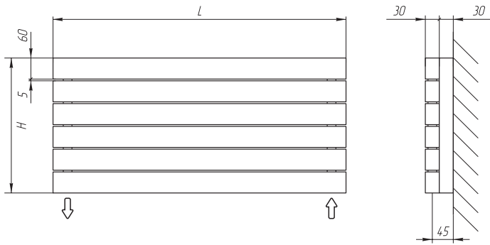
Нижнее подключение
