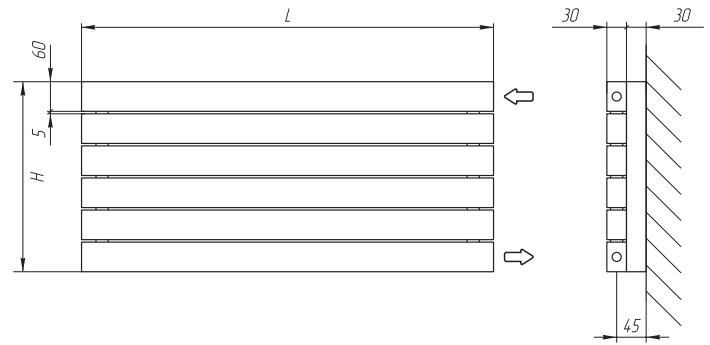
Боковое подключение
